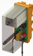
Brems-Chopper | Brake-Chopper 1415-0230
