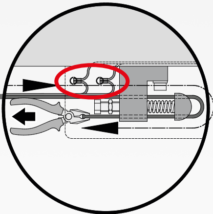
Torseite mit Spanneinheit Clamping unit
