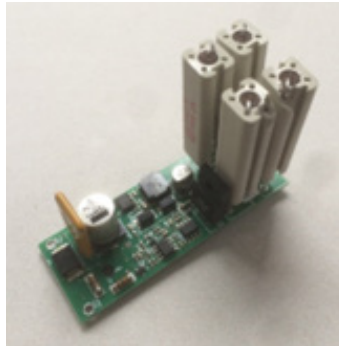
Bild 4 – Externer Brems-Chopper ohne Montagesockel
