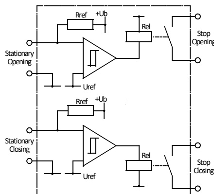
Prinzipschaltbild / Simplified diagram
